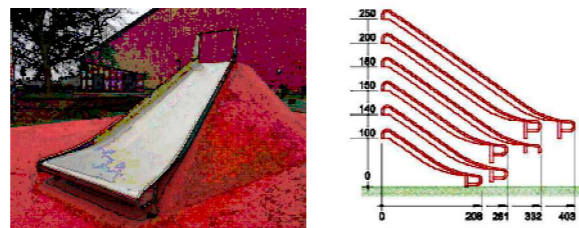
6. Tobogan doble d'acer inoxidable i plataforma de sortida de fusta; H 250 cm / Longitud 403 cm
